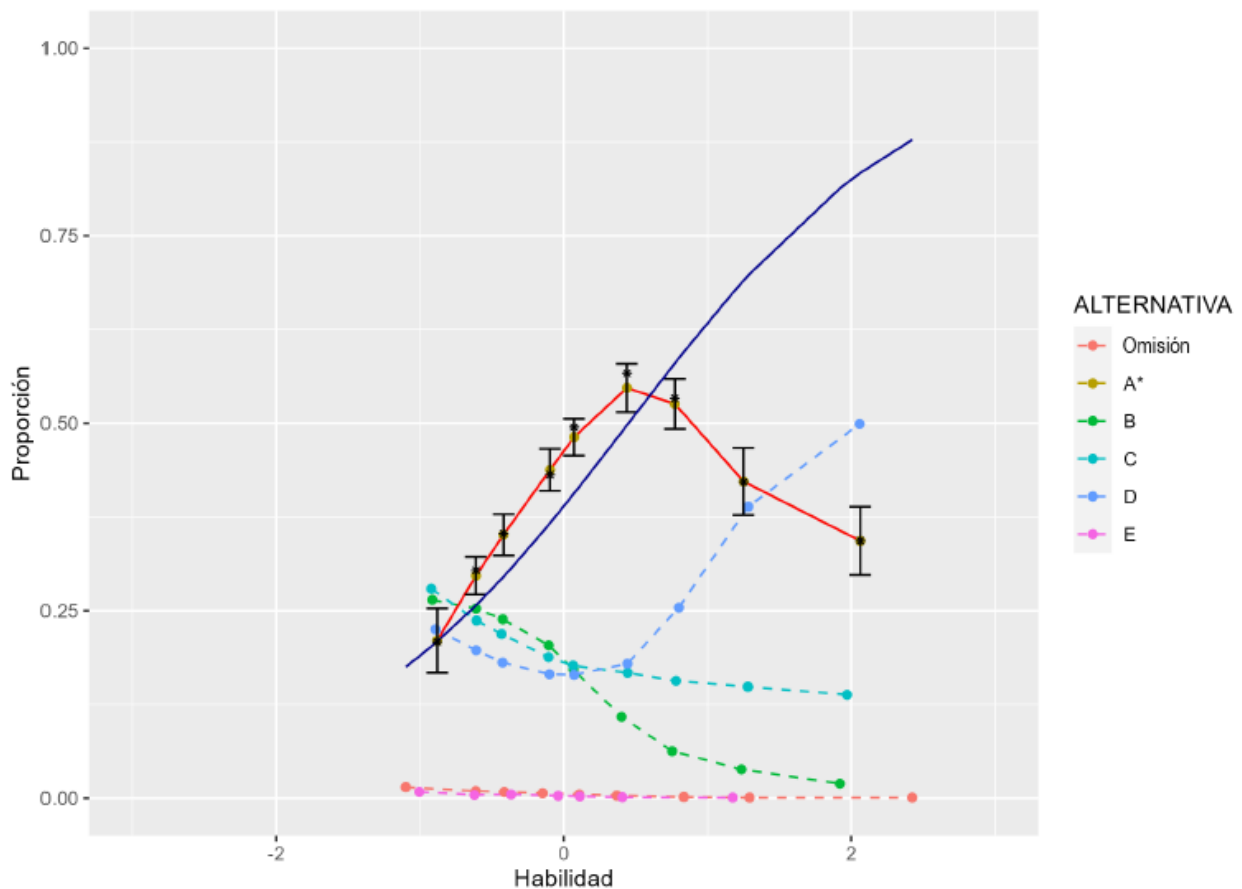
Figura 101: Ejemplo de curva característica de ítem, no creciente en todo el rango de habilidad
